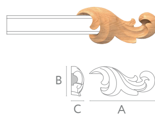
art. N.VRS-008R Наконечник на молдинг MLD-001
