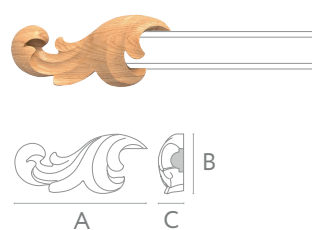
art. N.VRS-008L Наконечник на молдинг MLD-001
