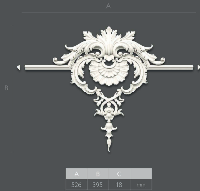
art. NPU-416.4 Накладка на молдинг MLDPU-004
