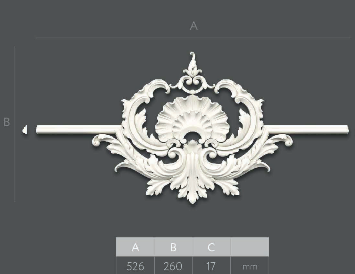
art. NPU-417.4 Накладка на молдинг MLDPU-004
